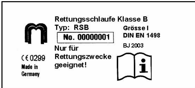
Bild 21: Muster der Kennzeichnung einer Rettungsschleufe
