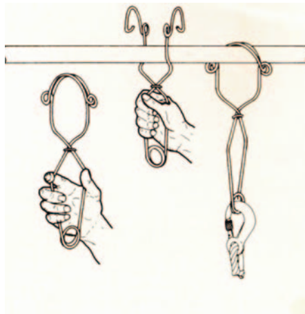
Bild 12: Anschlaghilfe
