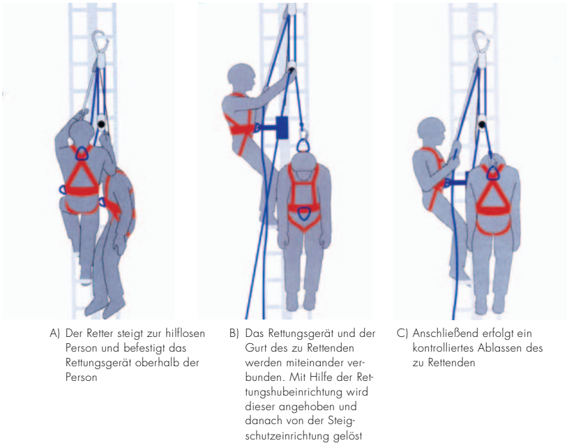
Bild 18: Rettung aus einer Steigschutzzeinrichtung mittels Abseilgerät, Rettungshubeinrichtung und Teleskopstange
