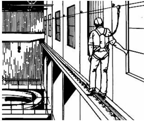
Bild 14: Anschlagereinrichtung mit horizontalem Führungsseil
