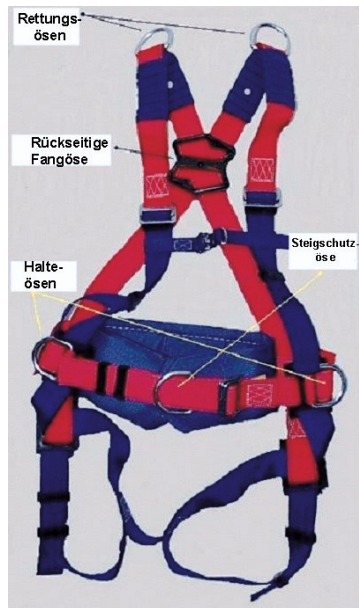
Bild 2: Rettungsgurt mit Polsterung der Gurtbänder
