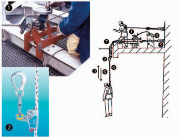
Bild 19: Rettung einer frei hängenden Person
