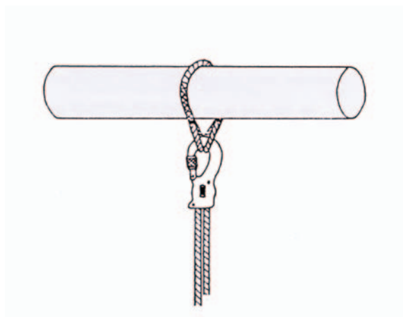
Bild 13: Anschlagseil mit zwei Augspießen
